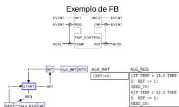
Exemplo de ECC e Algoritmo em um FB
