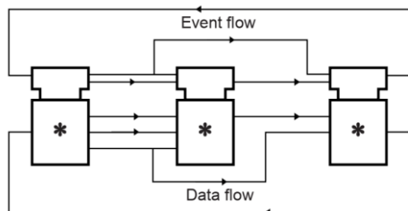
Modelo de Aplicação ( IEC61499-1:2013)
