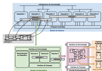
Visão geral dos modelos que compõem a IEC 61499 (Adaptado de Zotti 2008, Apud Leitão 2022)
